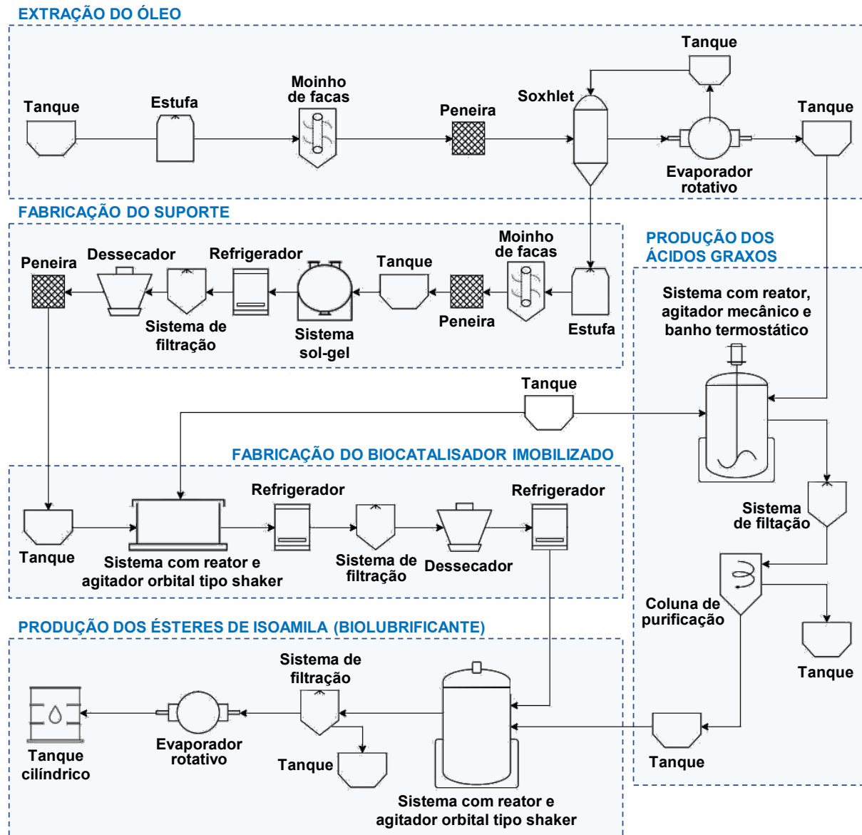
Figura 1 - Diagrama de fluxo do bioprocesso para valorização integral de sementes de Moringa oleifera Lam e produção de biolubrificante em escala de laboratório.
