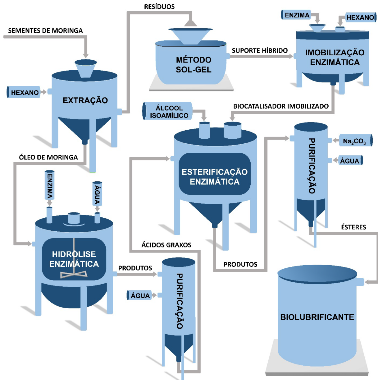
Figura 3 – Diagrama esquemático da unidade de bioprocesso integrado para a produção de biolubrificante.
